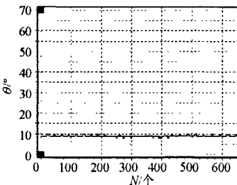
图 4 动态时由卡尔曼滤波计算的倾角
